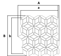
mod D A 52,9 cm - 20 7 / 8 " a 46,6 cm - 18 3 / 8 " B 54,2 cm - 21 1 / 8 " b 49,3 cm - 19 3 / 8 "
